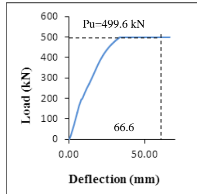
(b) FS300-16
